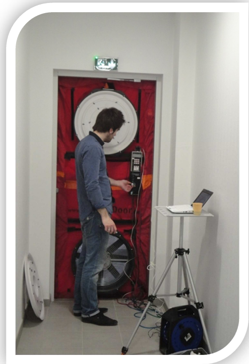
Test de la porte soufflante
